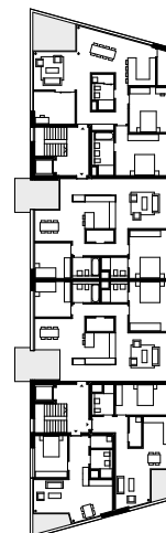
Obergeschoss
