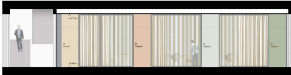
Schnitt B-B 1:50
