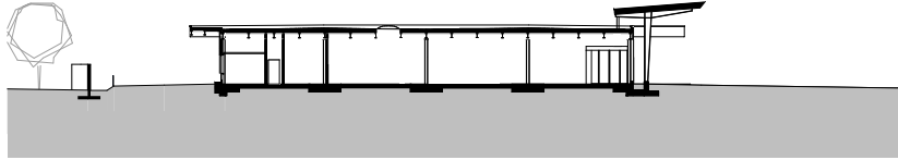
Querschnitt
